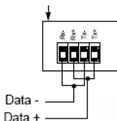
Рисунок 2 — Схема подключения по RS-485
