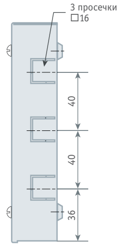
Вид справа
