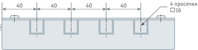
Вид снизу
